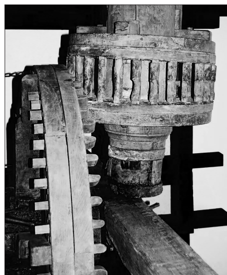
Зубчатые колёса. Фото из сети Интернет
